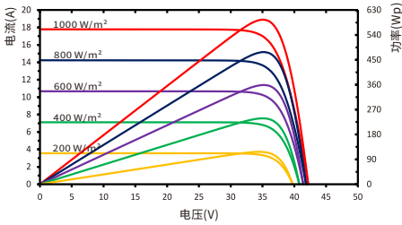
RSM110-8-595BHDG 不同辐照度下, I-V 曲线图
